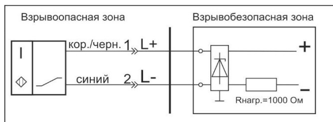
Схема соединения
