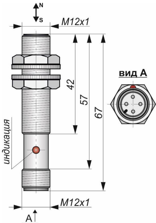
Габаритный чертеж
