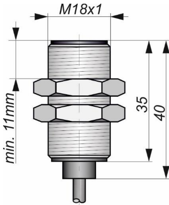
Габаритный чертеж
