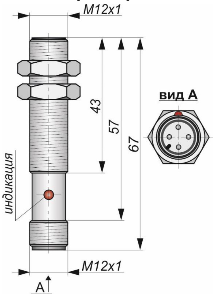
Габаритный чертеж
