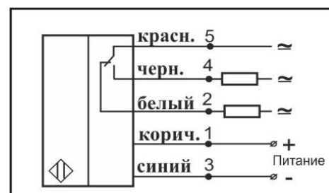
Схема соединения
