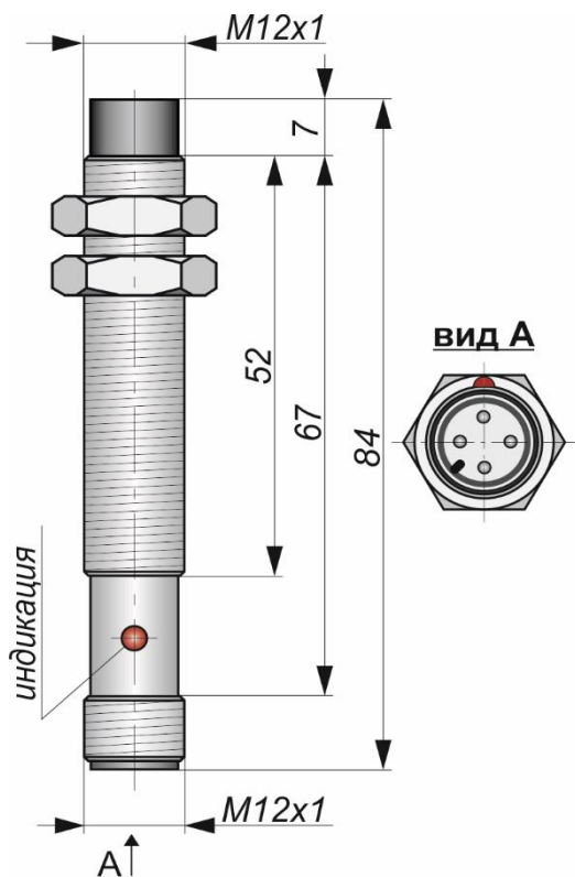
Габаритный чертеж
